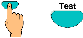
Abb. 42: Lampentest starten
