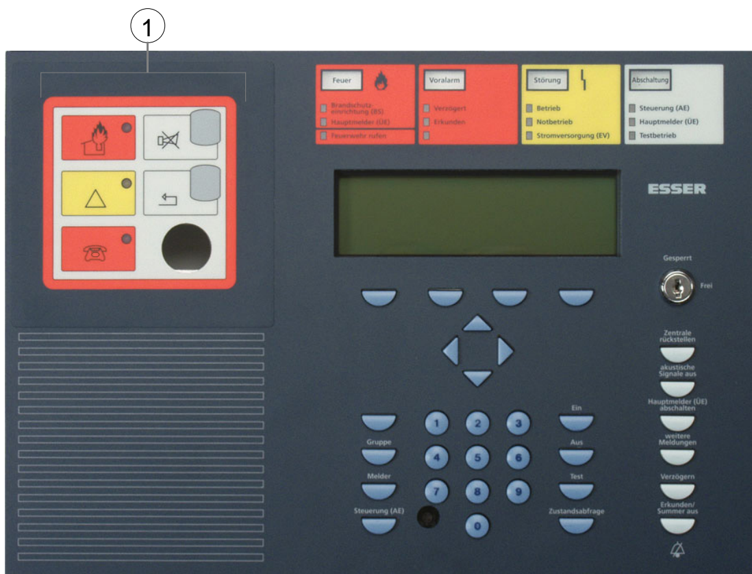
Abb. 10: Bedienteilfront mit integriertem Feuerwehrbedien- und Anzeigenteil (FBA)
