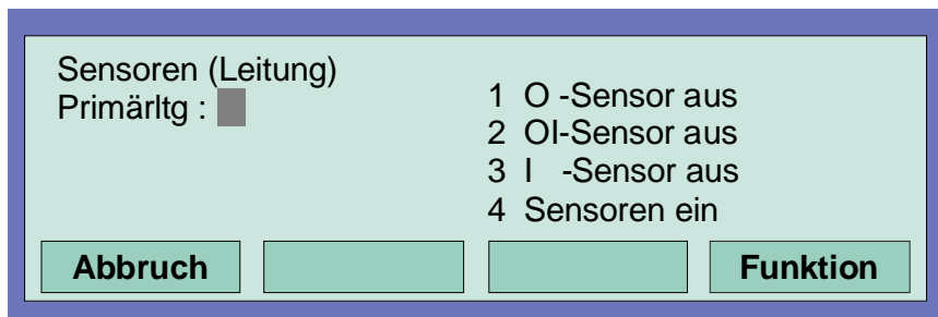
Abb. 47: Primärleitungsbezogene Sensorfunktionen
